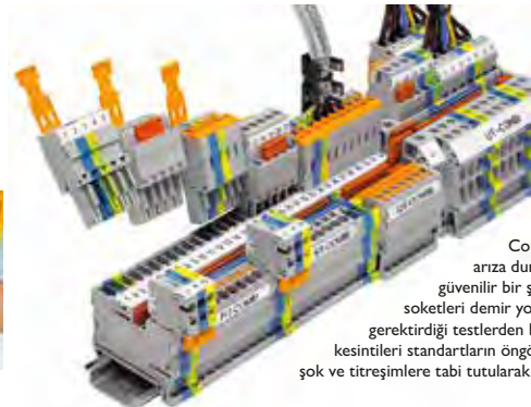
Vıdalı fişlerin kablo giriş yönü üstten veya yandan olabilir
