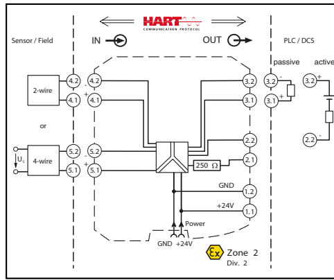
MACX MCR-SL-RPSSI-I için bağlantı şekli
