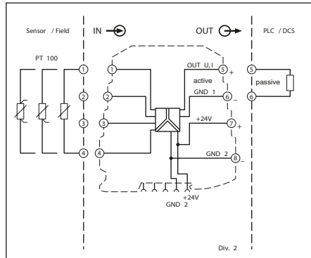
MINI MCR-SL-PT100-UI-NC için bağlantı şekli
