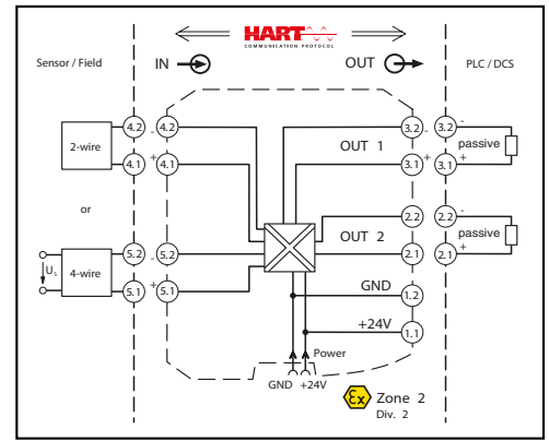
MACX MCR-SL-RPSSI-2I için bağlantı şekli
