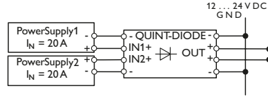
2 adet 20A güç kaynağının diyot modülüne bağlantısı
