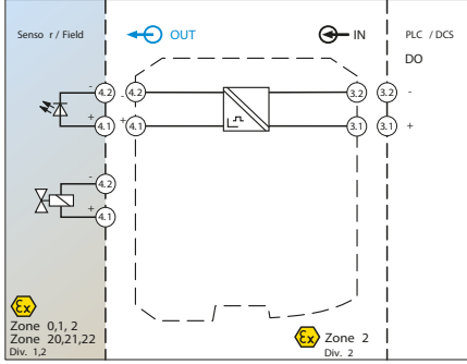
MACX MCR-EX-SL-SD-21-25-LP için bağlantı şekilleri
