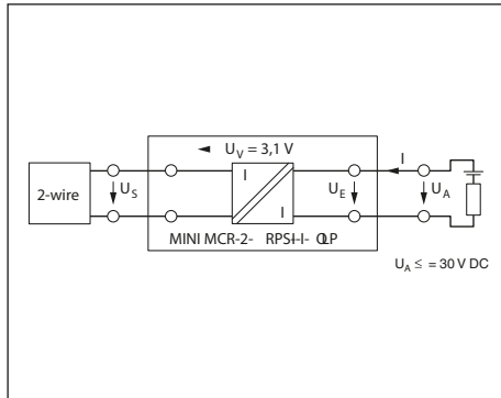
MINI MCR-2-RPS-I-I-OLP-PT için bağlantı şekli
