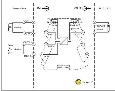
MINI MCR-2-UI-I-OLP-PT için bağlantı şekli
