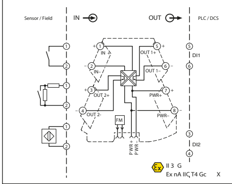
MINI MCR-2-NAM-2RO-PT için bağlantı şekli
