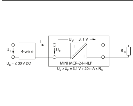
MINI MCR-2-I-I-ILP-PT için bağlantı şekli
