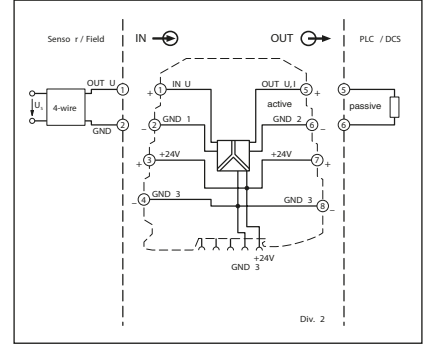
MINI MCR-SL-UI-UI-NC için bağlantı şekli
