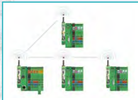
I/O bilgisinin Modbus RTU formatında iletilmesi
