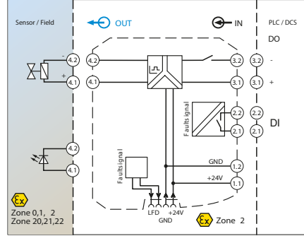
MACX MCR EX-SL-23-48-LFD için bağlantı şekilleri
