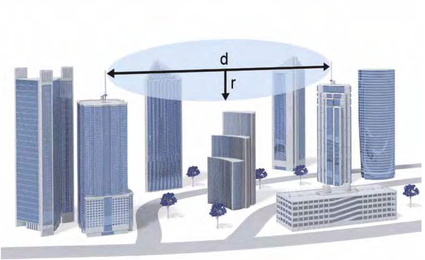
Şekil : Fresnel-Zone
