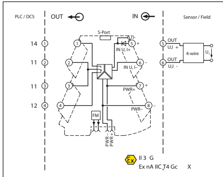
MINI MCR-2-UI-REL-PT için bağlantı şekli
